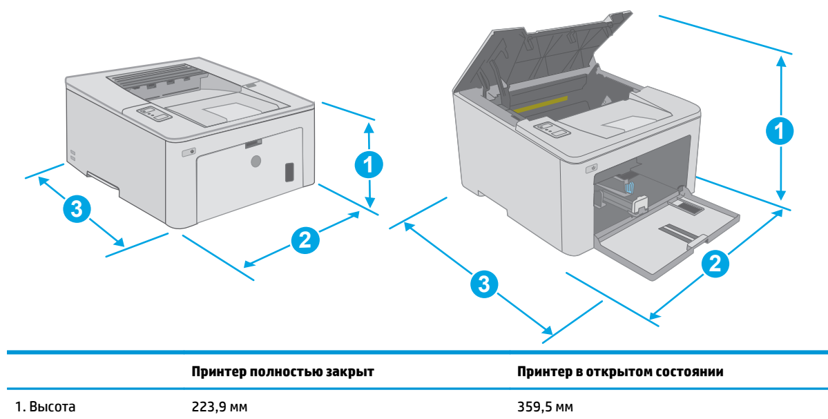
Рисунок 1-1 Размеры принтера
