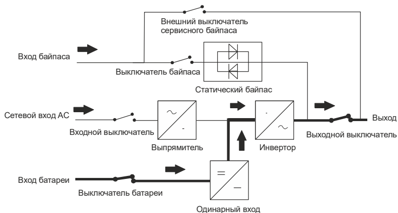
Рисунок 19 - Режим работы «РЕЗЕРВ» с раздельным вводом байпас
