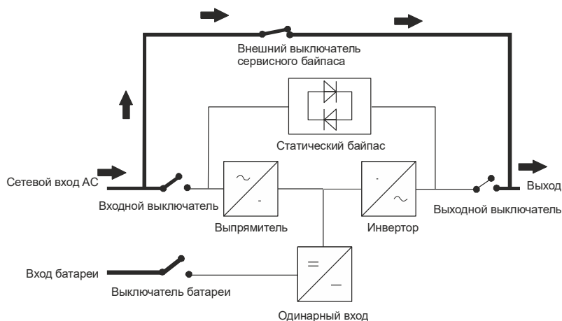
Рисунок 24 - Режим работы ручной байпас с одиночным вводом питания
