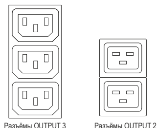
Рисунок 30 Разъемы сегментов OUTPUT 3 и OUTPUT 2
