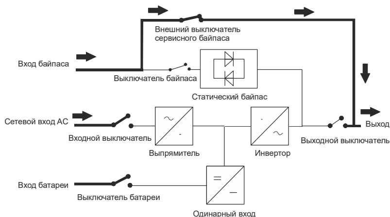
Рисунок 25 - Режим работы ручной байпас с разделенным вводом байпаса
