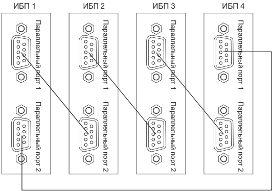
Рисунок 14 - Схема подключения кабеля параллельной работы
