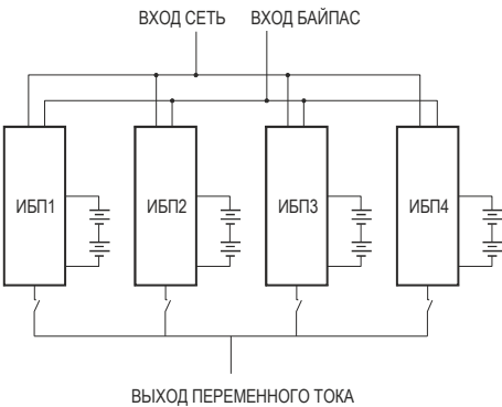
Рисунок 12 –Схема с отдельным вводом байпас
