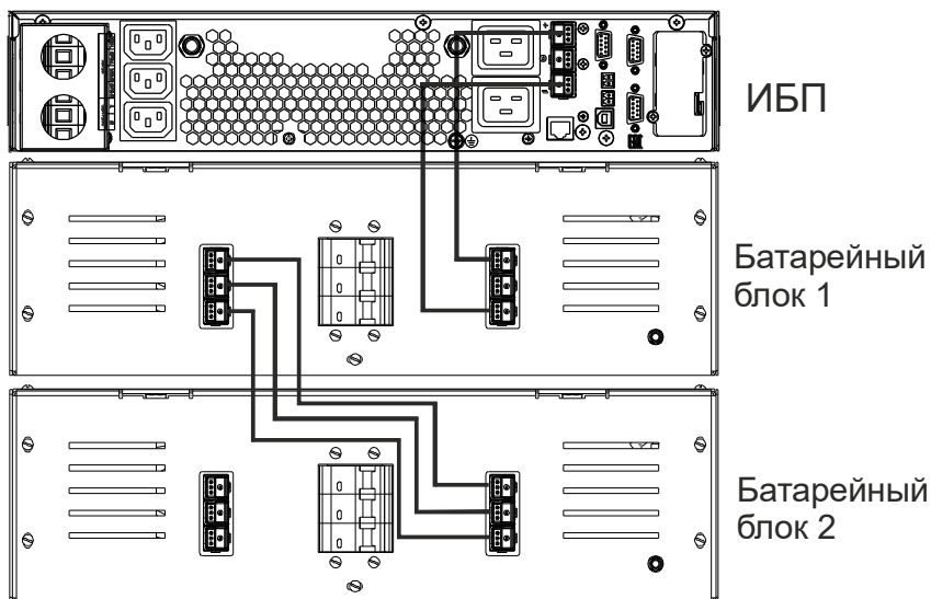
Рисунок 10 – Схема подключения нескольких внешних батарейных блоков (кабель, соединяющий между собой батарейные блоки, входят в комплект поставки батарейных блоков)
