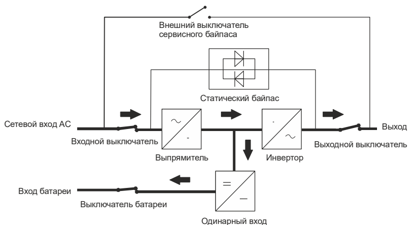
Рисунок 17 - Режим работы «ОСНОВНОЙ» с раздельным вводом байпас
