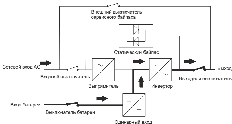
Рисунок 18 - Режим работы «РЕЗЕРВ» с одиночным вводом питания
