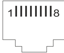
Рисунок 34 - Назначение контактов RS-485 порта
