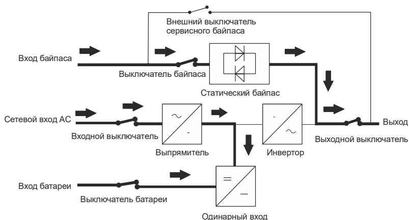
Рисунок 21 - Режим работы «БАЙПАС» с отдельным вводом байпас
