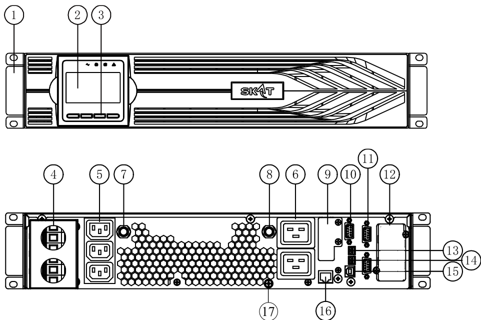
Рисунок 2 – Общий вид передней и задней панели SKAT-UPS 6000-RACK-ON P3, SKAT-UPS 10000-RACK-ON P3
