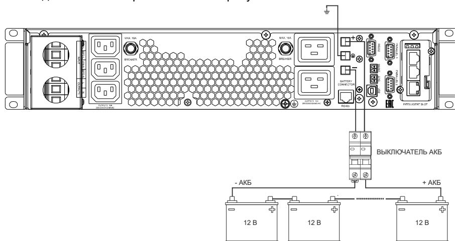
Рисунок 9 – Подключение внешних батарей
