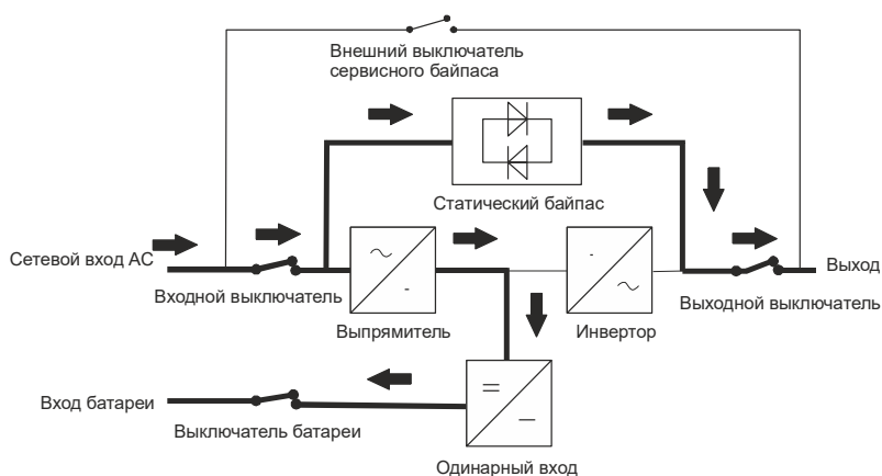
Рисунок 20 - Режим работы «БАЙПАС» с одиночным вводом питания
