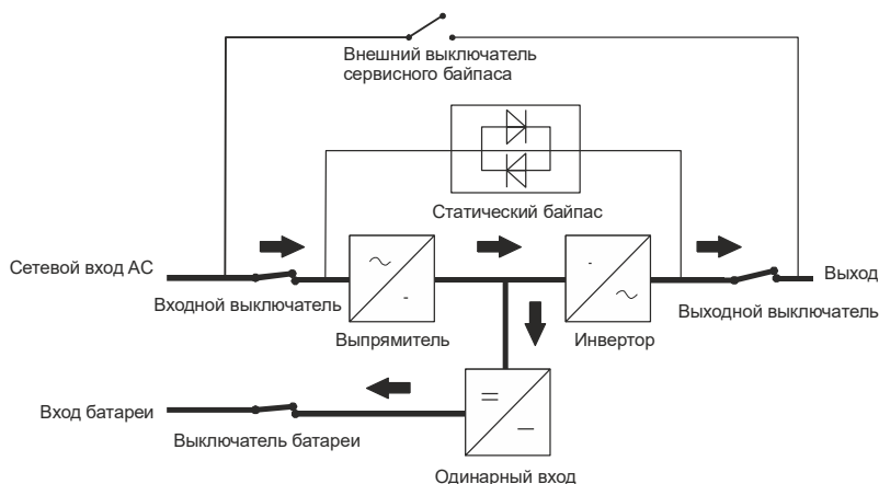
Рисунок 16 - Режим работы «ОСНОВНОЙ» с одиночным вводом питания
