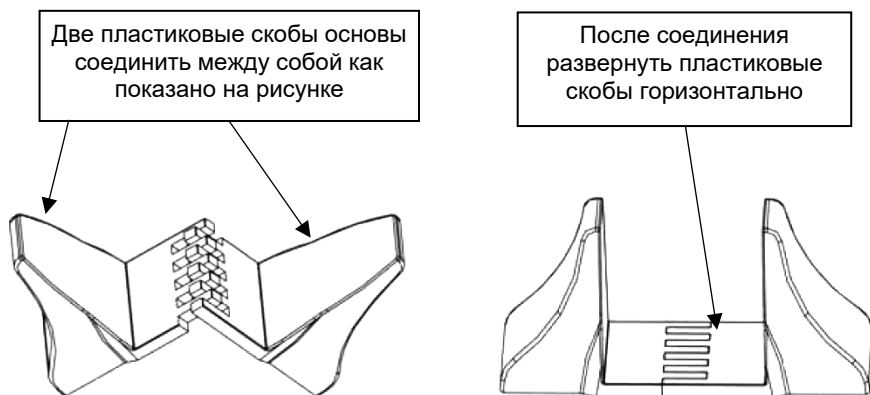
Рисунок 5 – Сборка основы из пластиковых подставок
