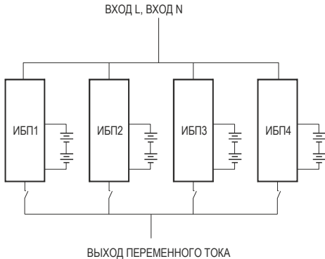
Рисунок 13 –Схема с единым вводом питания
