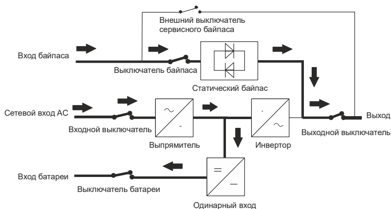
Рисунок 23 - Режим работы ECO с разделным вводом байпас
