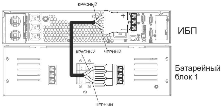
Рисунок 11 – Кабель для подключения внешнего батарейного блока
