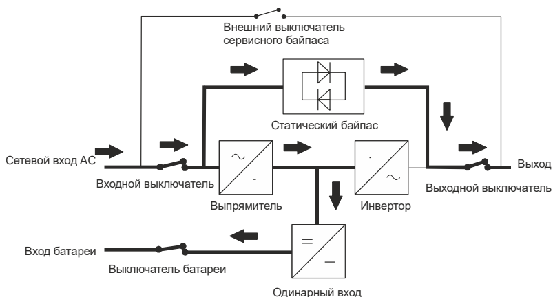
Рисунок 22 - Режим работы ECO с одиночным вводом питания
