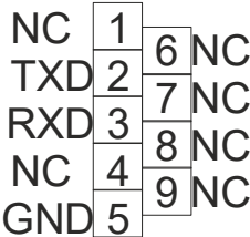
Рисунок 33 - Назначение контактов RS-232 порта
