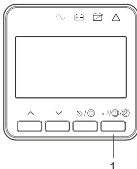
Рисунок 26 - Кнопка включения ИБП в режиме «Холодный старт».
