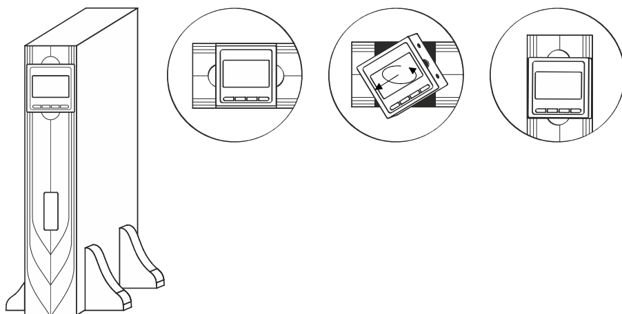
Рисунок 6 – Поворот ЖК-дисплея при напольной установке
