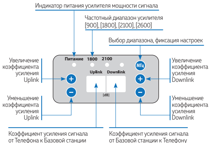
Рисунок 6 – элементы панели управления усилителя мощности сигнала
