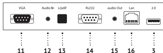
Нижняя панель
