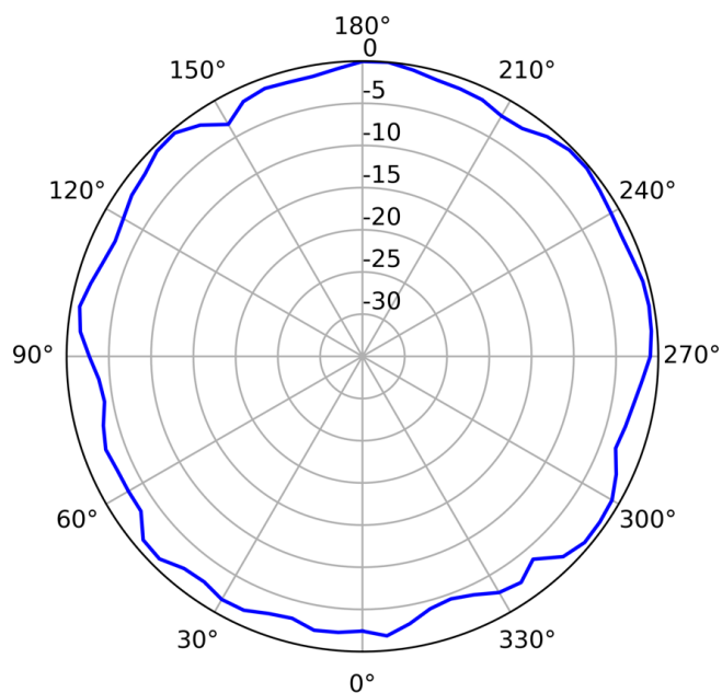
5GHz (Horizontal)
