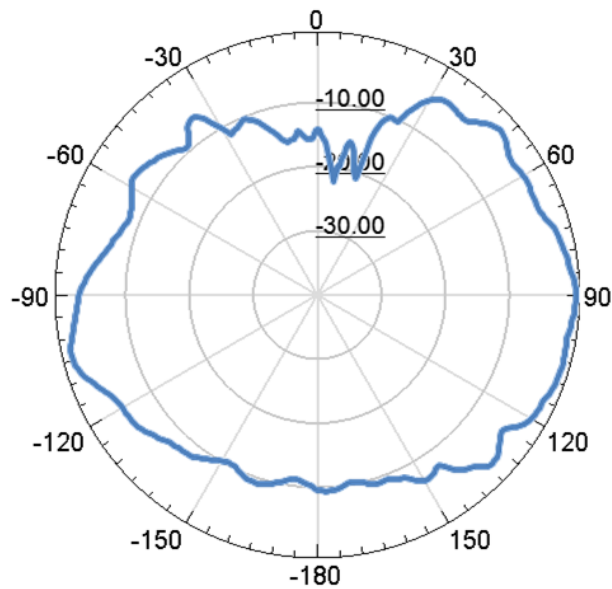
5GHz (Vertical)
