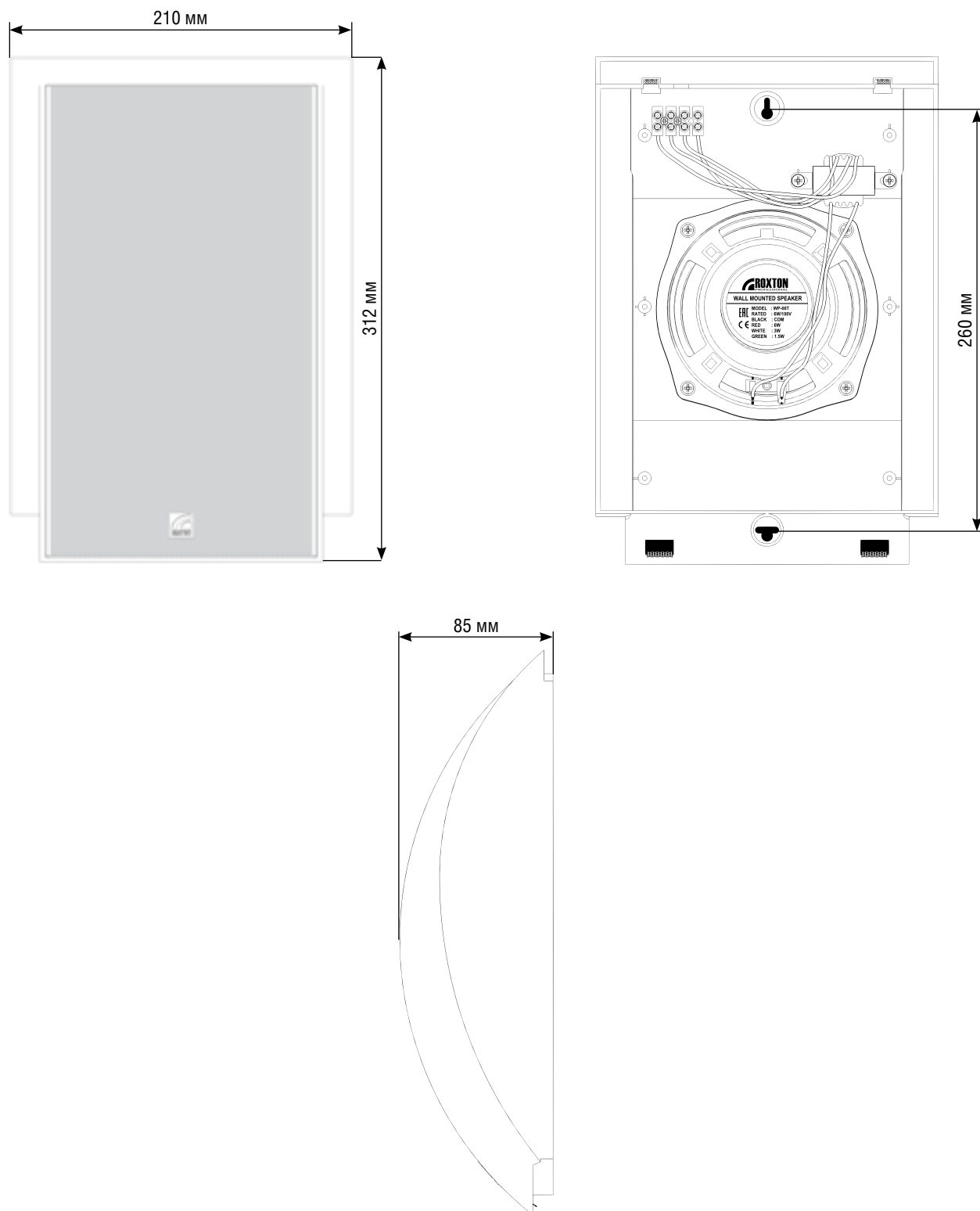
Рисунок А.1 Габаритные размеры ROXTON WP-06T
