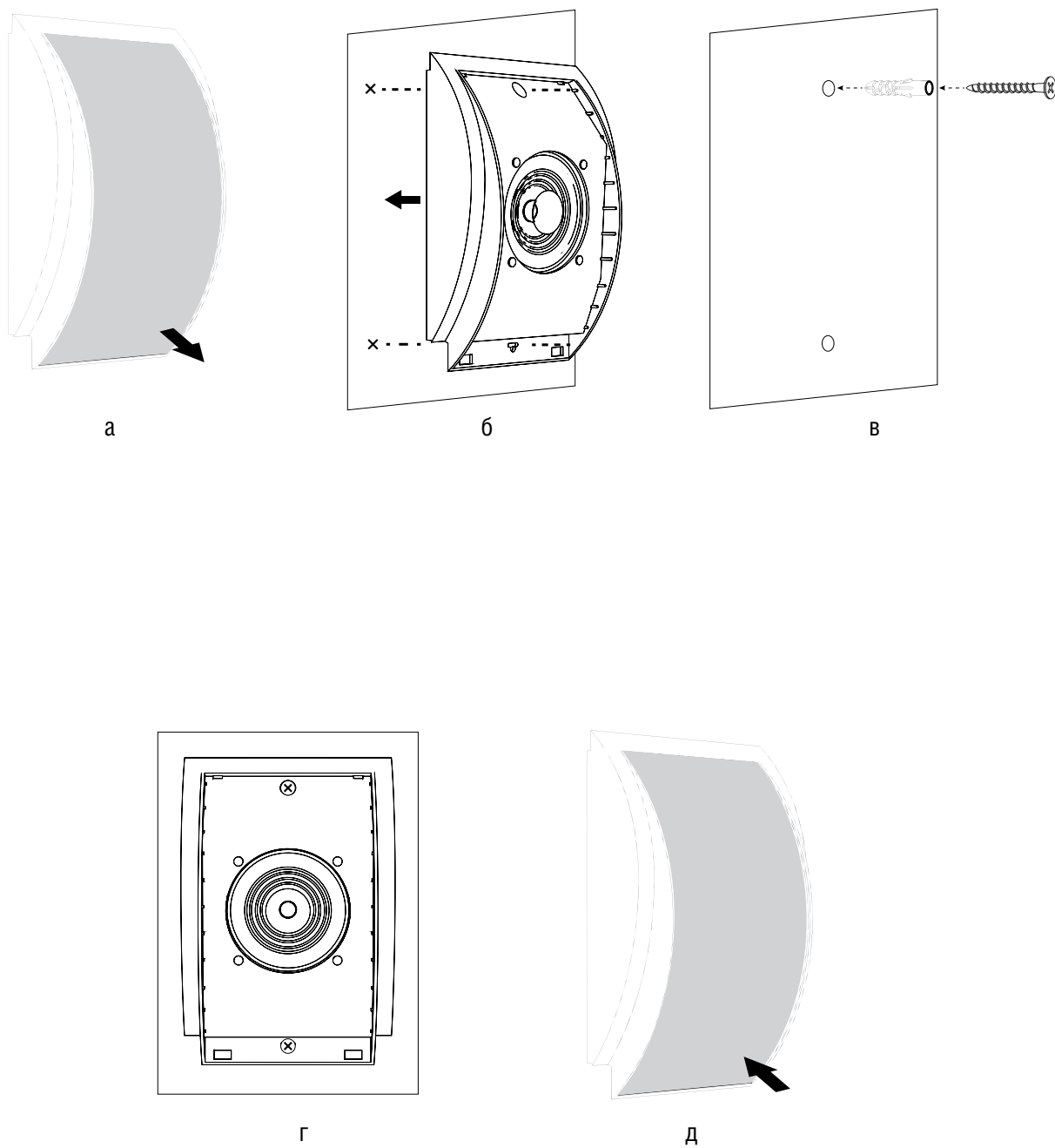
Рисунок 7.2 Порядок установки громкоговорителя
