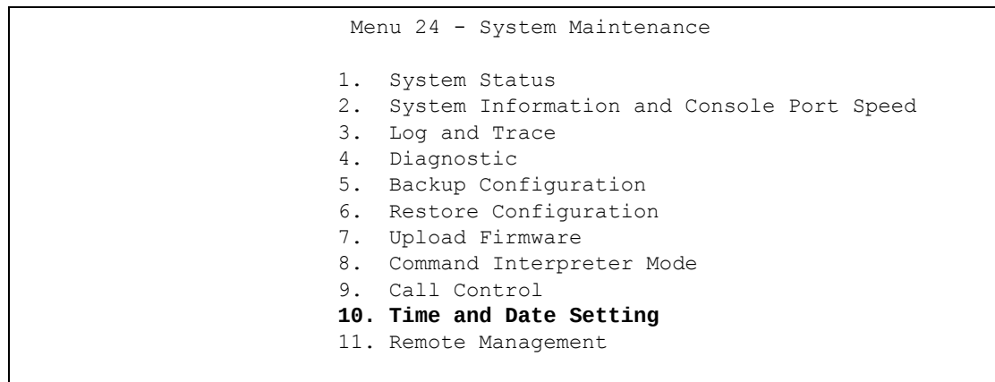
Рис. 234 Меню 24: Обслуживание системы
