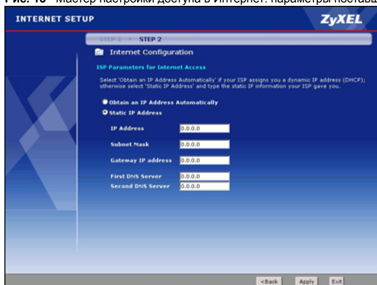
Рис. 13 Мастер настройки доступа в Интернет: параметры поставщика услуг Интернета (Ethernet)
