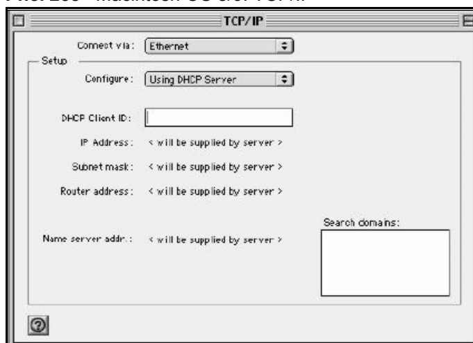
Рис. 258 Macintosh OS 8/9: TCP/IP
