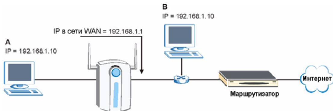
Рис. 283 Конфликты IP-адресов: случай С
