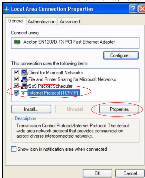
Рис. 253 Windows XP: Свойства подключения по локальной сети
