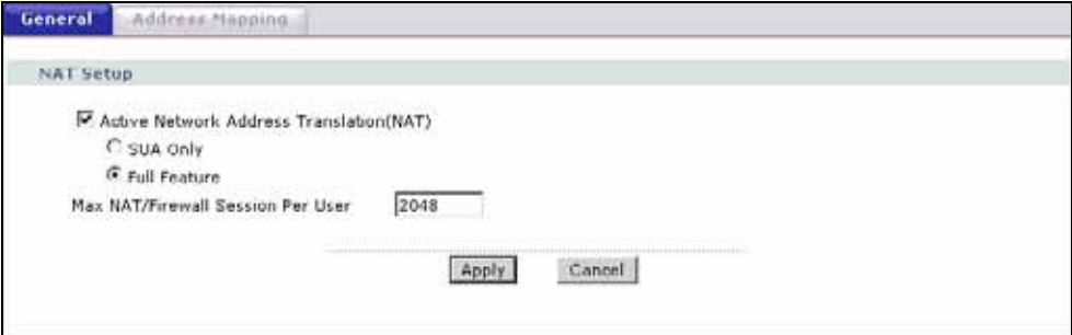
Рис. 46 Экран NAT > General
