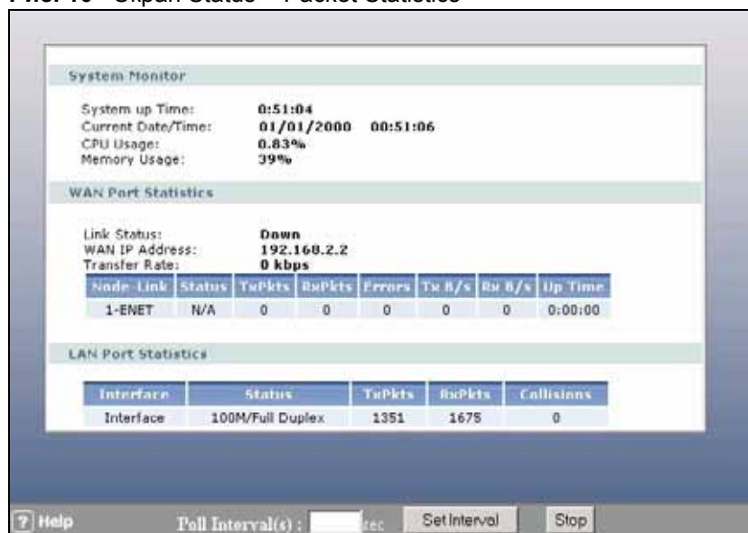
Рис. 10 Экран Status > Packet Statistics
