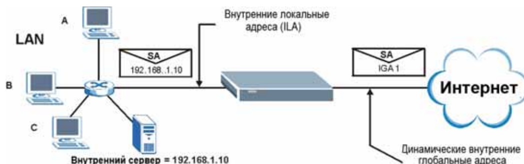
Рис. 174 NAT: пример 2
