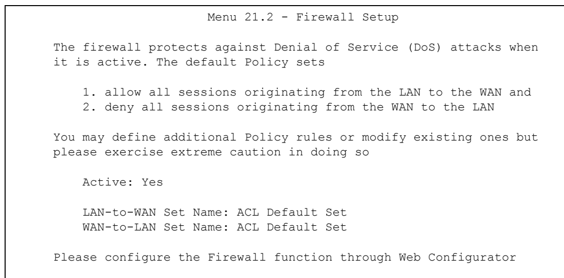
Рис. 185 Меню 21.2: Настройка межсетевого экрана
