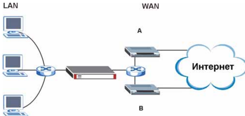
Рис. 288 Резервный шлюз
