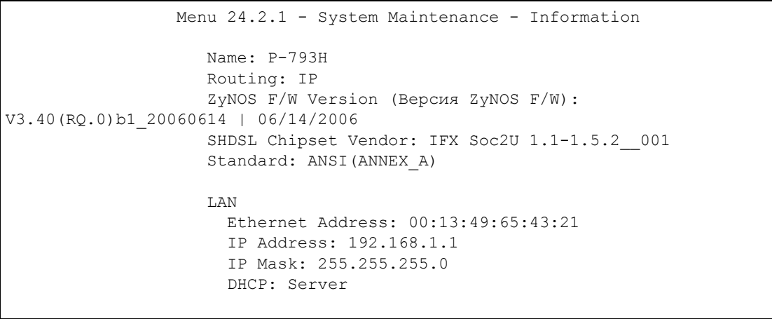
Рис. 205 Меню 24.2.1: Обслуживание системы – информация
