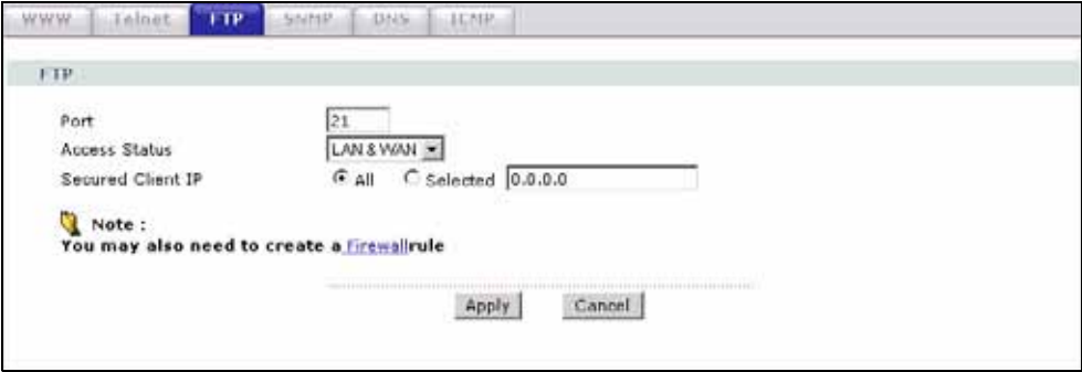
Рис. 102 Экран Remote MGMT > FTP
