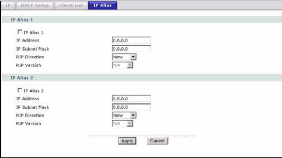
Рис. 43 Экран LAN > IP Alias
