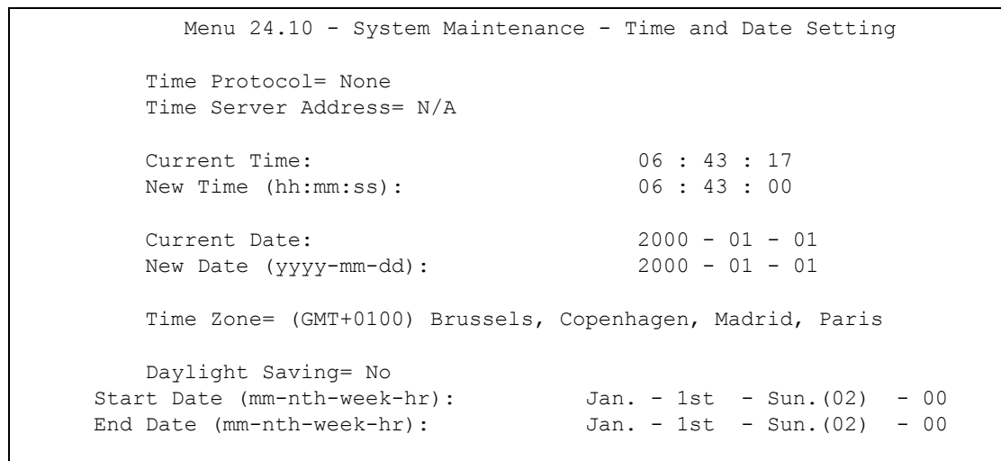
Рис. 235 Меню 24.10: Управление системой – настройка времени и даты
