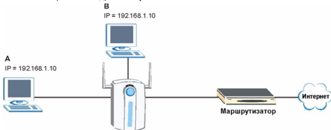
Рис. 284 Конфликты IP-адресов: случай D
