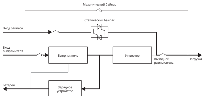
Рис 2-6 Блок-схема Экономичного режима
