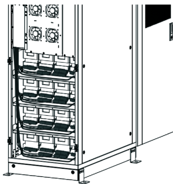
Рис 6-5 Установка защитной панели клеммного терминала подключения батарей
