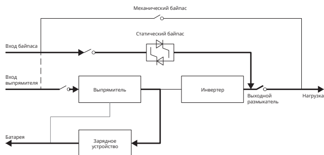
Рис 2-4 Блок-схема Режим байпаса
