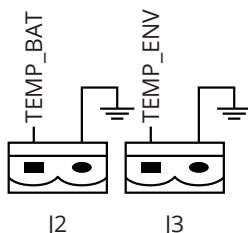
Рис 3-14 Контакты J2 и J3 для измерения температуры
