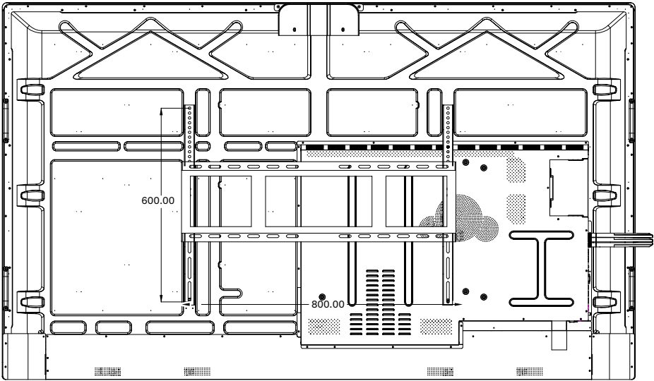
СХЕМА ДИСПЛЕЯ (ВИД СЗАДИ)
