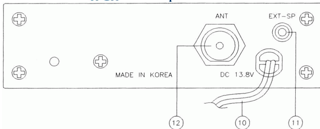
Рис. 2 Органы управления и отображения MJ-300
