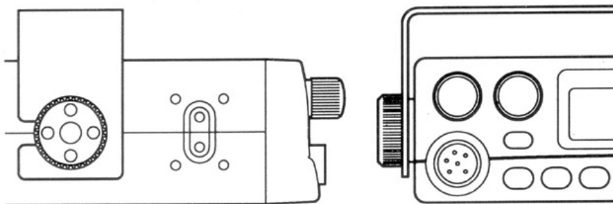
Рис. 4. Крепление радиостанции фиксаторами.
