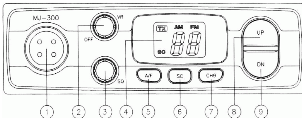
Рис. 1. Органы управления и отображения MJ-300
