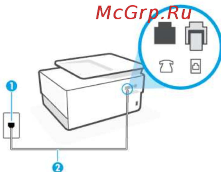
Рисунок 9-1 Вид принтера сзади
