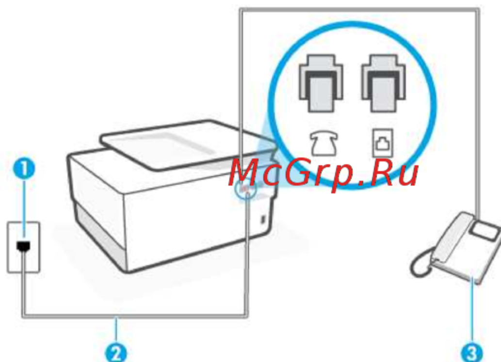
Рисунок 4-4 Вид принтера сзади
