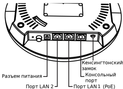
Рис. 2 Задняя панель DWL-7620AP
