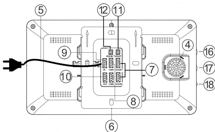
Конструкция монитора
