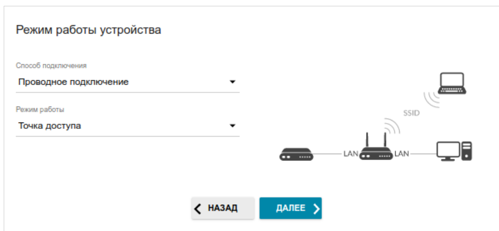
Рисунок 35. Выбор режима работы устройства. Режим Точка доступа .
