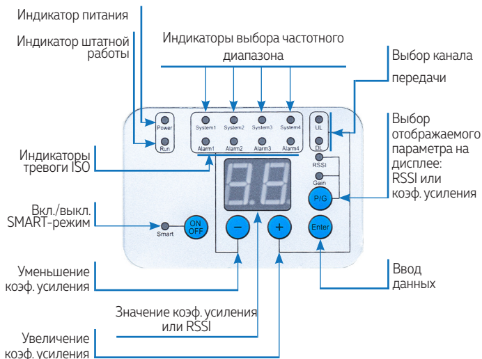
Рисунок 5 – элементы панели управления усилителя мощности сигнала
