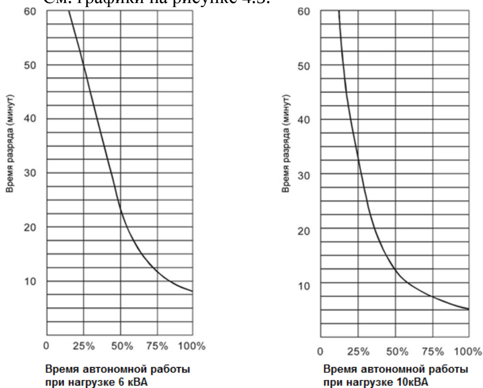
Рисунок 4.5 - Время автономной работы для стандартных ИБП
