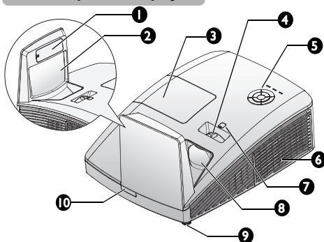
Вид спереди/сверху
