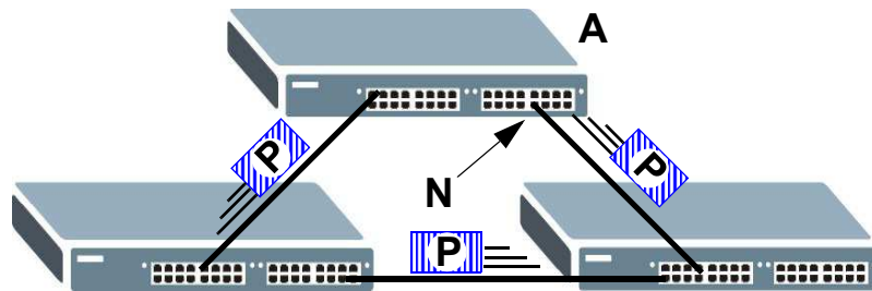
Рисунок 166 Защита от образования петель – петля в сети
