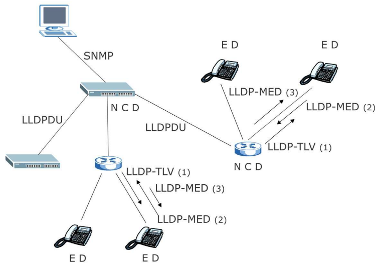
Рисунок 185 Обзор LLDP-MED
