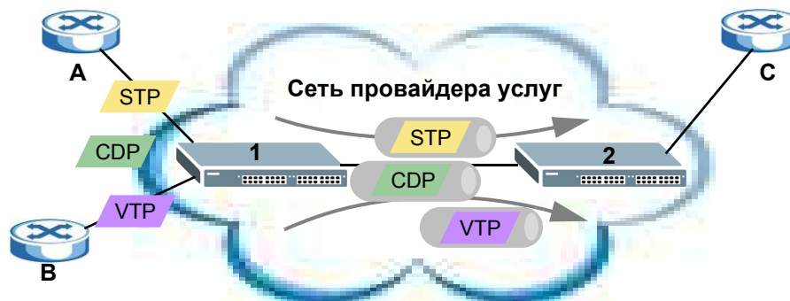
Рисунок 168 Сетевой сценарий туннелирования протоколов уровня 2
