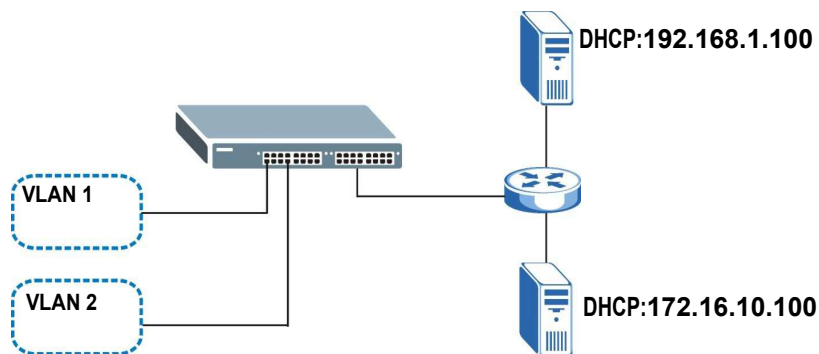
Рисунок 216 Ретрансляция DHCP для двух VLAN
