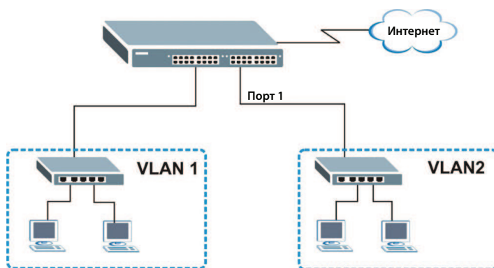
Рисунок 28 Пример первичной настройки сети: виртуальная локальная сеть
