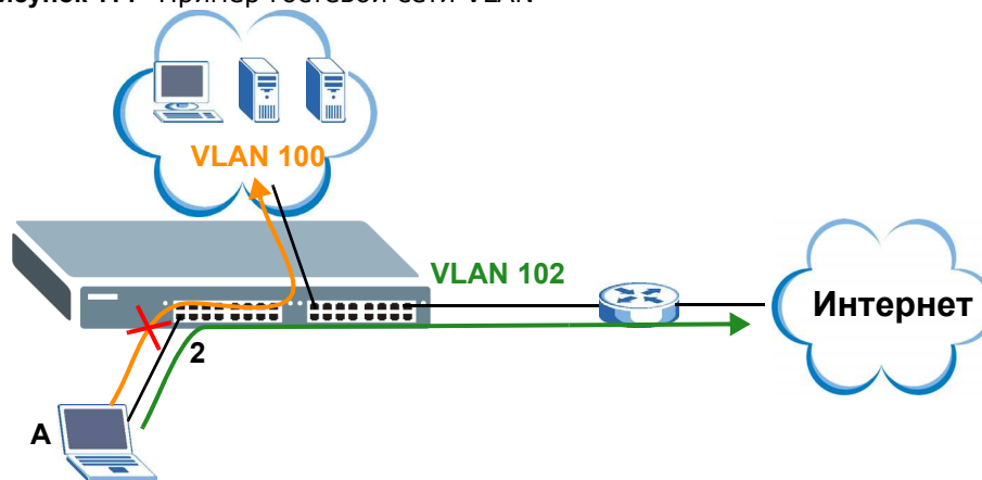
Рисунок 114 Пример гостевой сети VLAN
