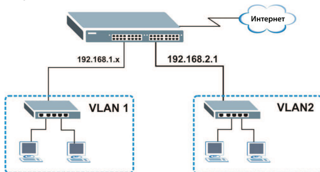
Рисунок 30 Пример первичной настройки: IP-адрес управления
