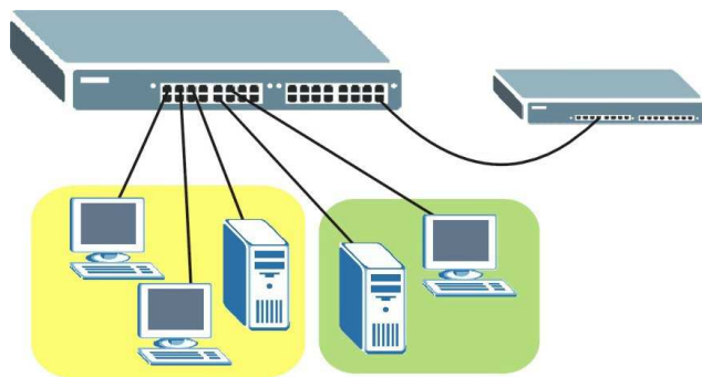
Рисунок 76 Пример использования VLAN на основе протоколов
