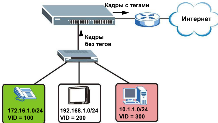
Рисунок 74 Пример использования VLAN на основе подсетей
