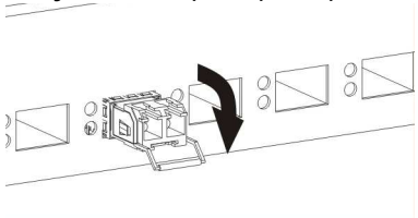
Рисунок 19 Пример удаления трансивера
