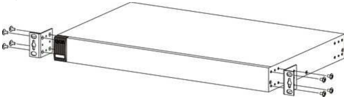
Рисунок 5 Закрепление кронштейнов
