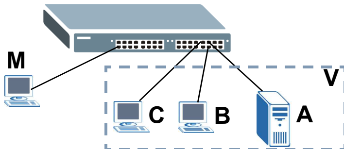
Рисунок 31 Пошаговые указания: Обзор пошаговых указаний по работе с функцией отслеживания DHCP
