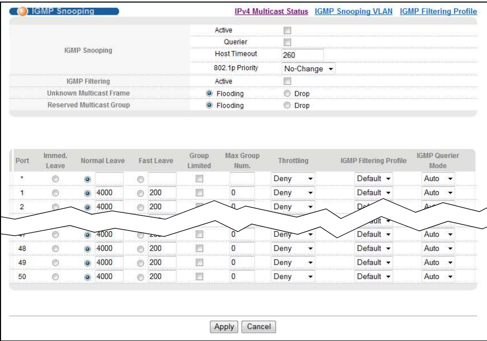
Рисунок 128 Экран Advanced Application > Multicast > IPv4 Multicast > IGMP Snooping
