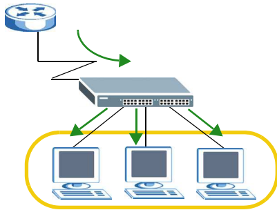
Рисунок 85 Многоадресная рассылка на основе статических адресов на один порт A
