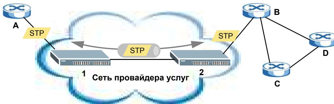
Рисунок 169 Пример сети с использованием L2PT
