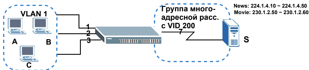
Рисунок 139 Пример настройки MVR
