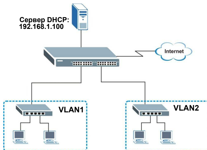
Рисунок 212 Пример сети с глобальной ретрансляцией DHCP
