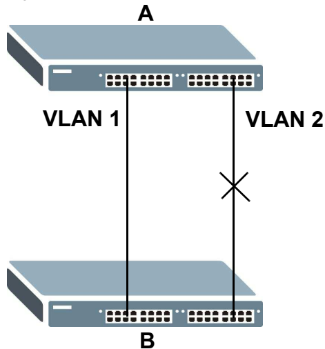
Рисунок 99 Пример сети с поддержкой STP/RSTP
