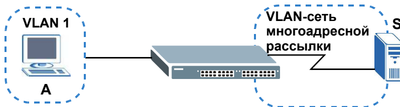
Рисунок 125 Пример с многоадресной рассылкой телевидения посредством MVR
