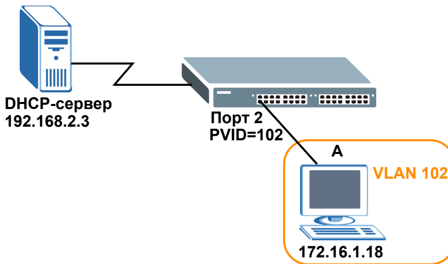
Рисунок 38 Пошаговые указания: Сценарий ретрансляции DHCP
