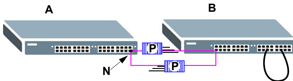
Рисунок 165 Защита от образования петель – пробный пакет
