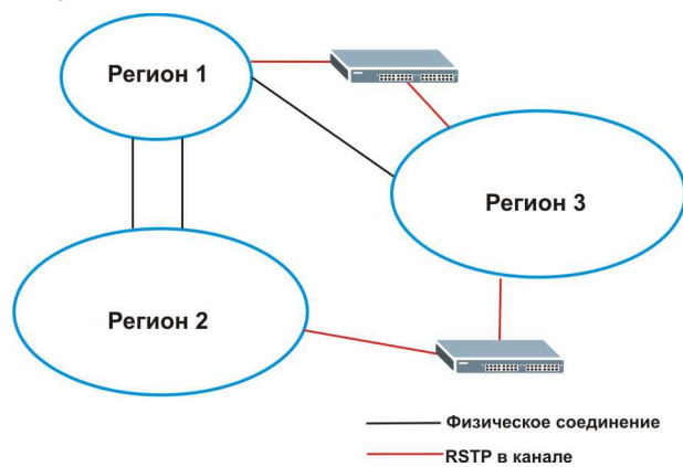
Рисунок 102 Пример сети с использованием MSTP и традиционного протокола RSTP
