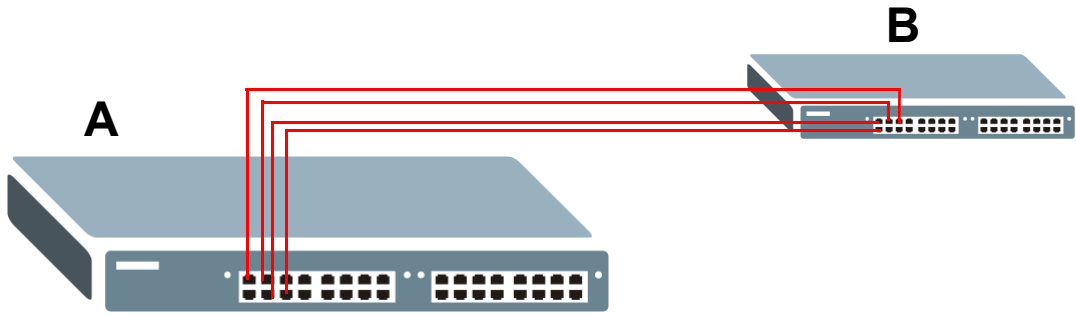
Рисунок 109 Пример группирования портов – физические подключения
