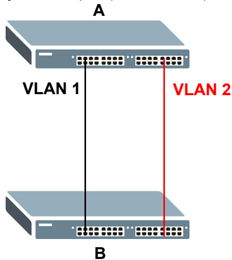
Рисунок 100 Пример сети с поддержкой MSTP
