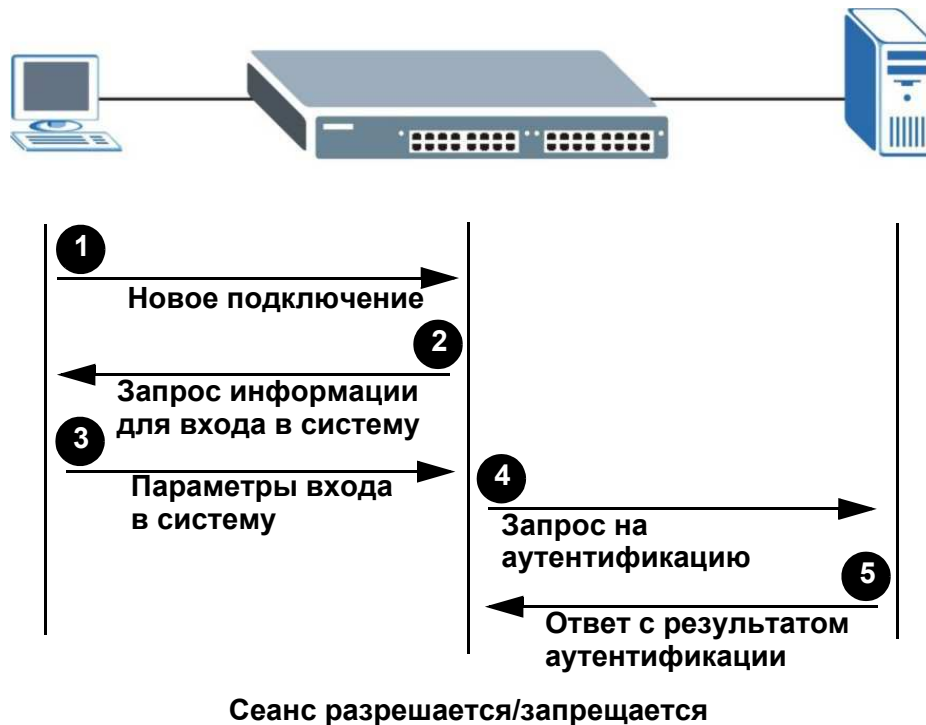
Рисунок 111 Процесс аутентификации на основе IEEE 802.1x
