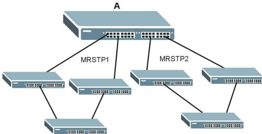
Рисунок 89 Пример сети с поддержкой MRSTP
