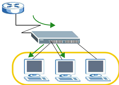
Рисунок 86 Многоадресная рассылка на основе статических адресов на два и более портов
