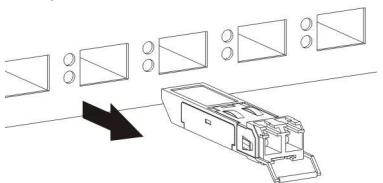
Рисунок 19 Пример удаления трансивера
