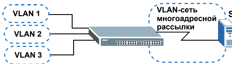
Рисунок 124 Пример сети с поддержкой MVR
