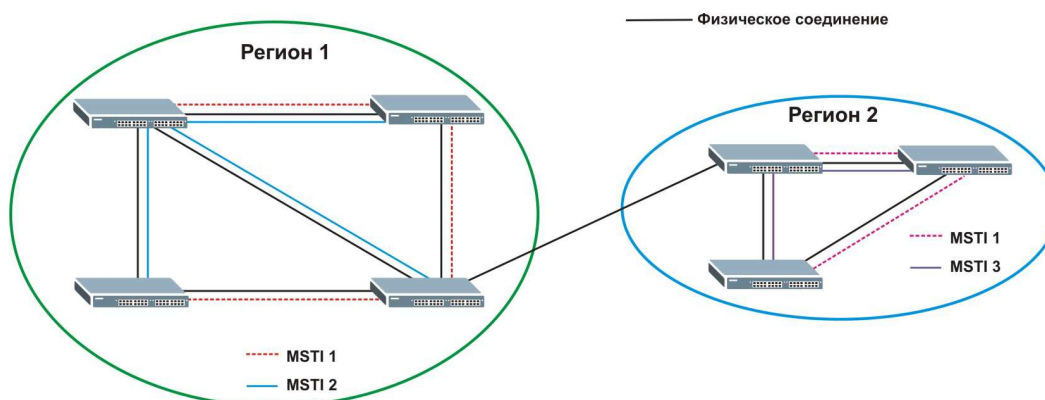
Рисунок 101 Экземпляры MSTI в различных регионах
