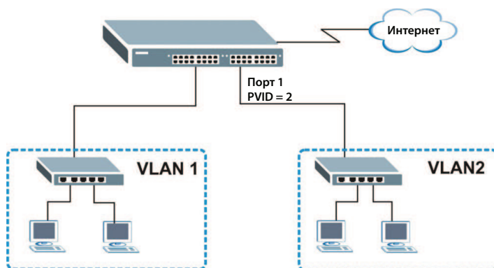
Рисунок 29 Пример первичной настройки сети: идентификатор виртуальной локальной сети для порта
