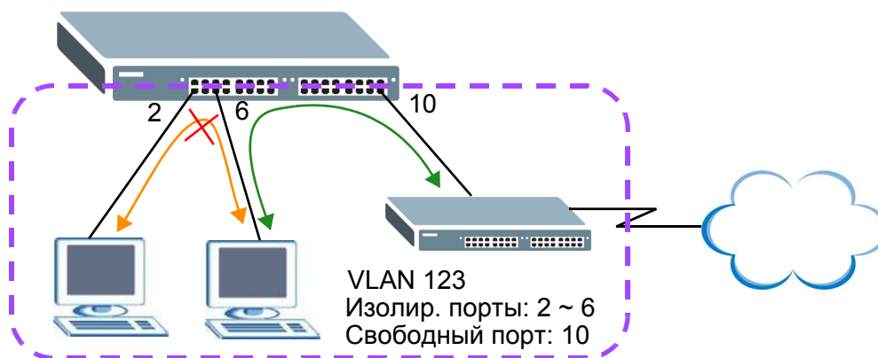
Рисунок 181 Пример частной сети VLAN
