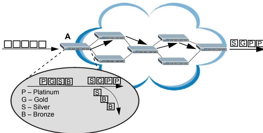
Рисунок 204 Сеть с поддержкой DiffServ
