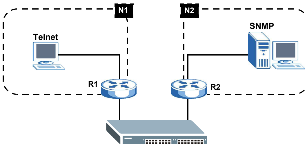
Рисунок 200 Обзор статических маршрутов
