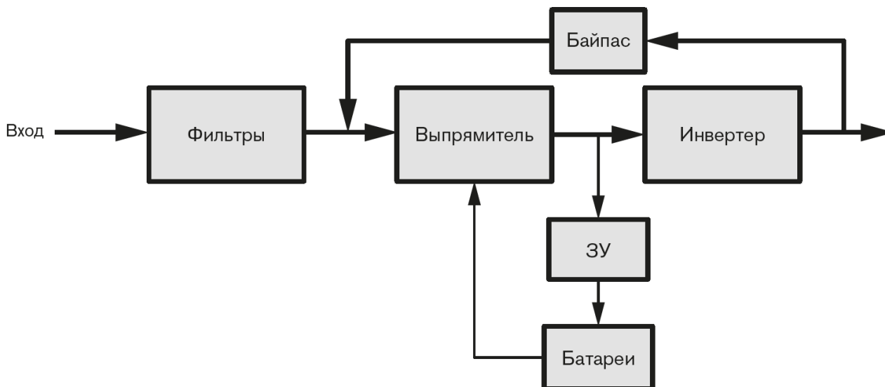
Рис. 3-6 Режим самодиагностики
