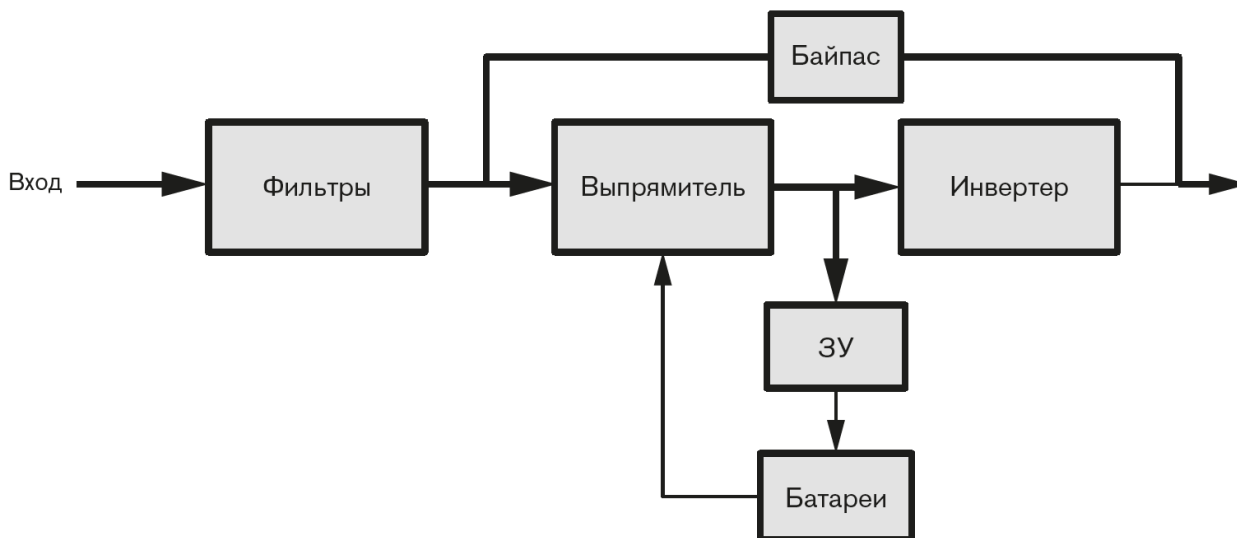
Рис. 3-5 ЭКО режим
